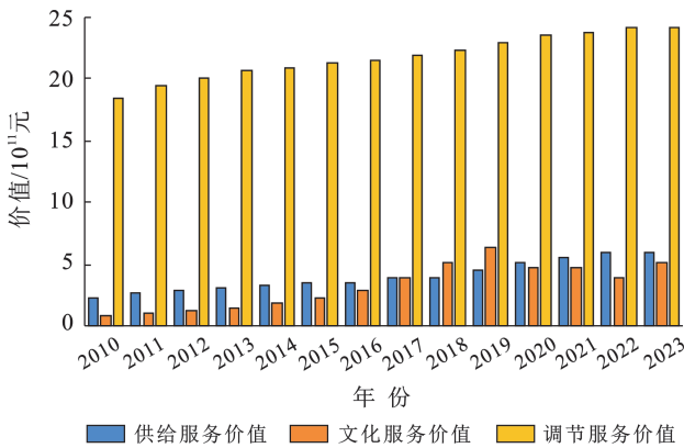
图 3 南岭民族走廊 2010—2023 年生态产品的供给服务价值、调节服务价值和文化服务价值
